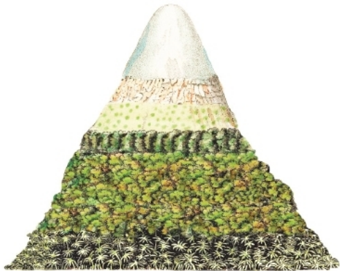
Representação esquemática do vulcão Chimborazo
